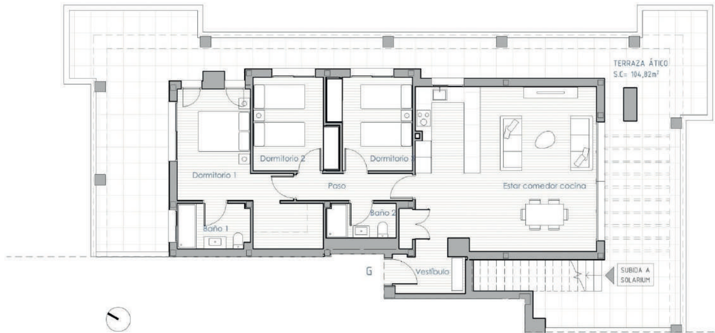
Planta ático
